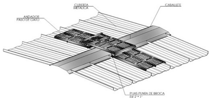
ISOMÉTRICO
