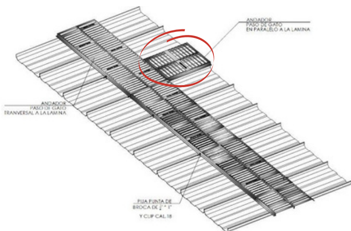
ISOMÉTRICO
