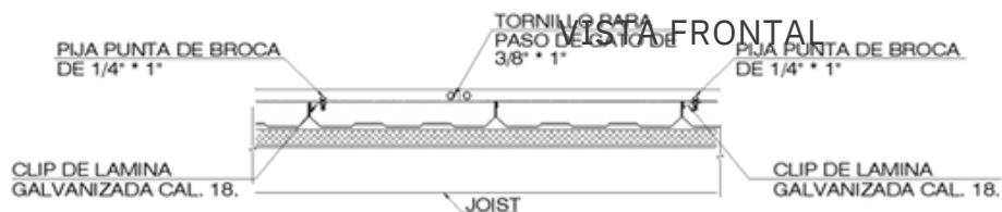
VISTA LATERAL
